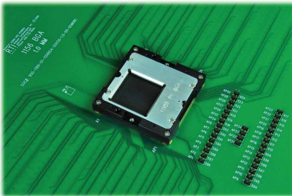
34x34 BGA Array
